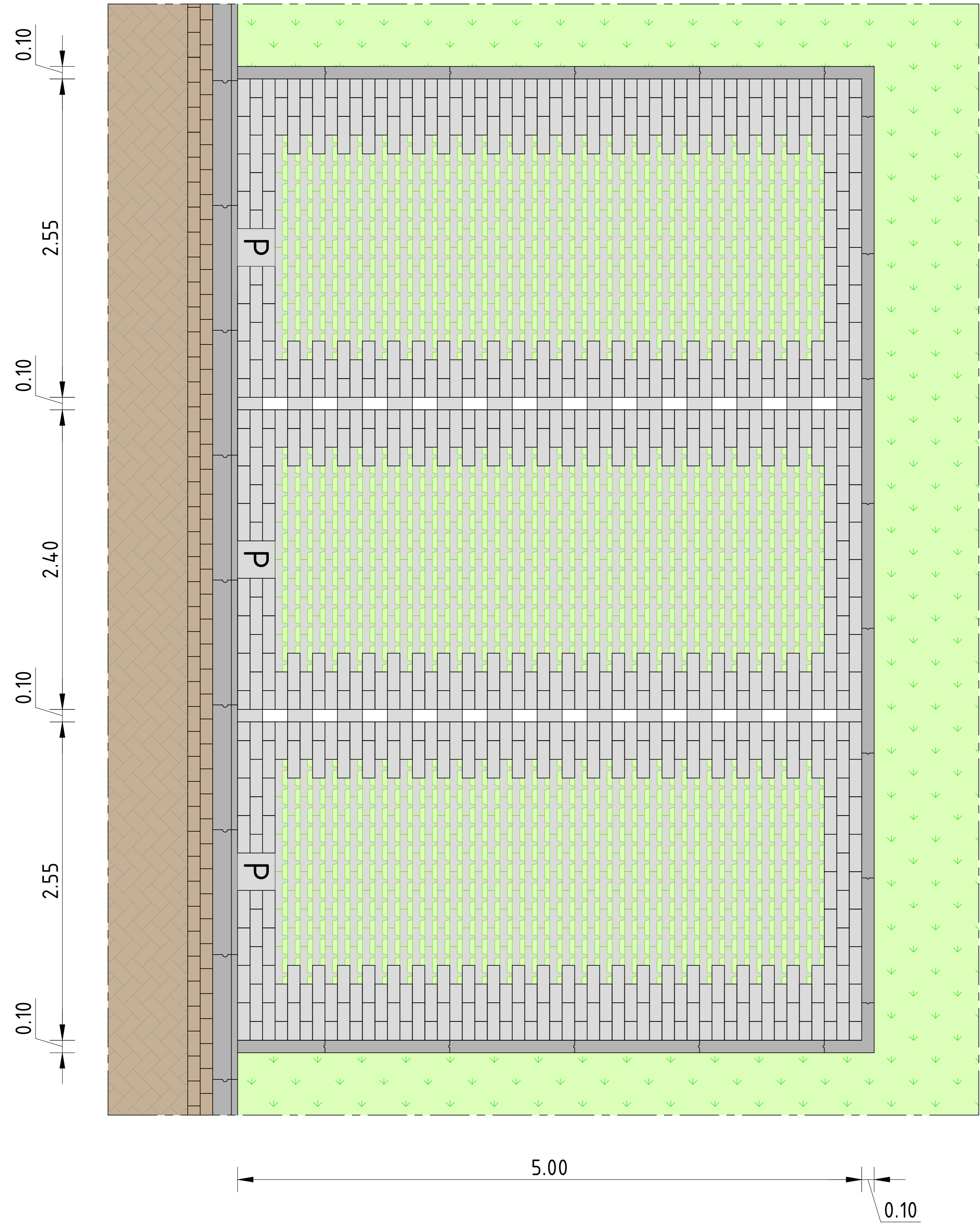
Principe detail haaks parkeervaak Schaal 1:20
