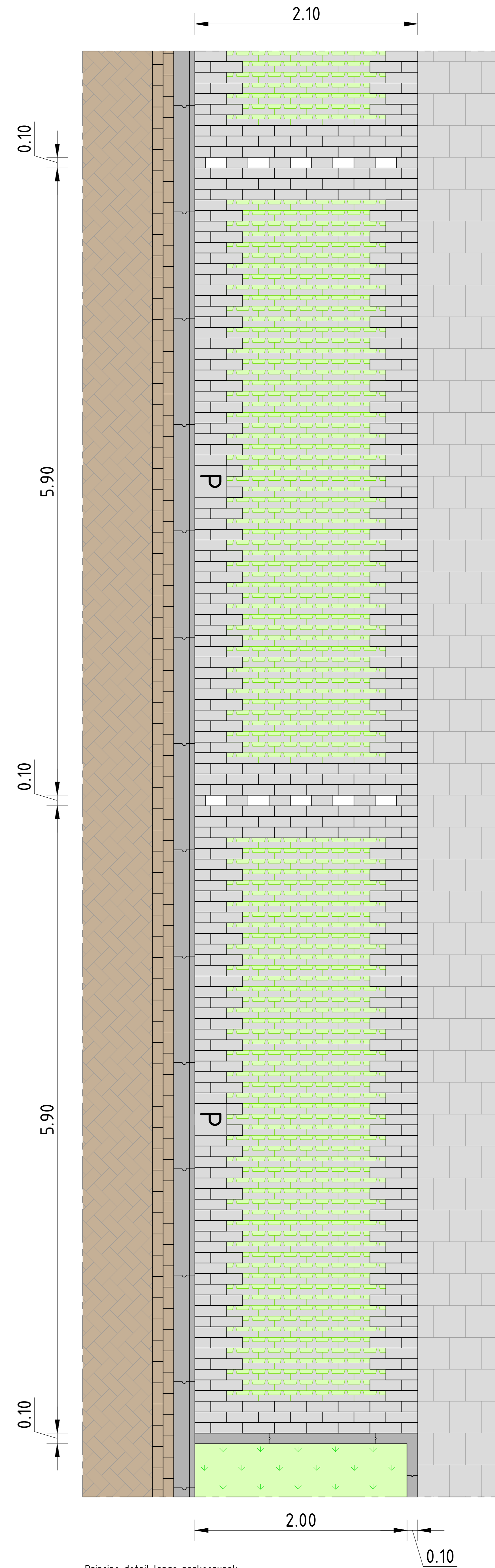
Principe detail langs parkeervaak Schaal 1:20
